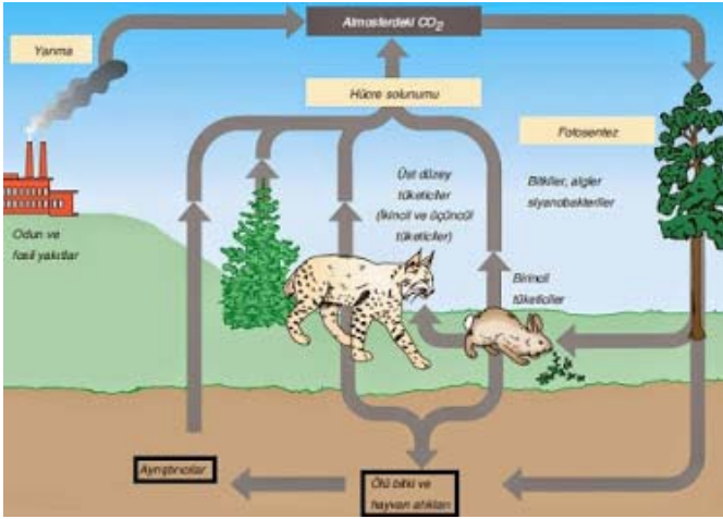
Karbon Döngüsü
