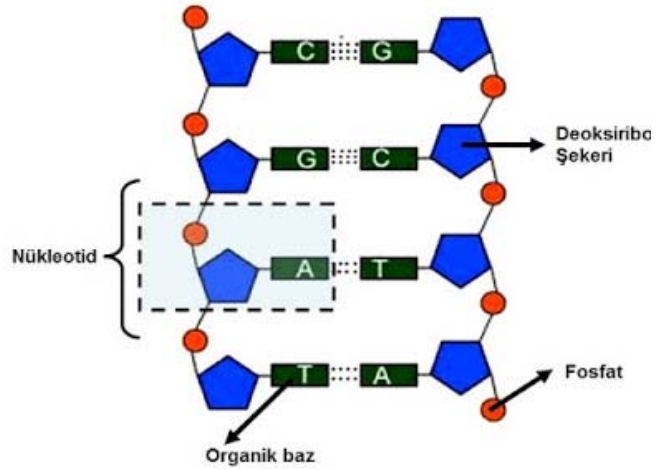
DNA Zinciri
